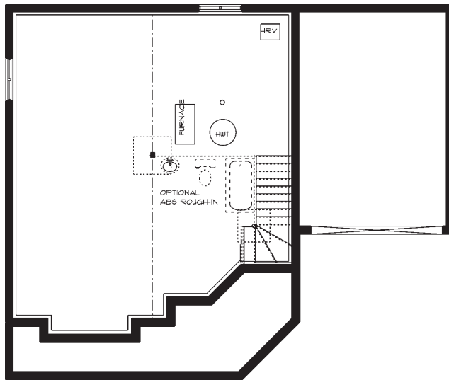
BASEMENT PLAN PLAN DU SOUS-SOL
