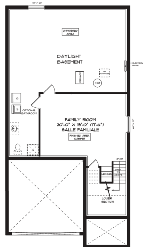
BASEMENT PLAN PLAN DU SOUS-SOL
