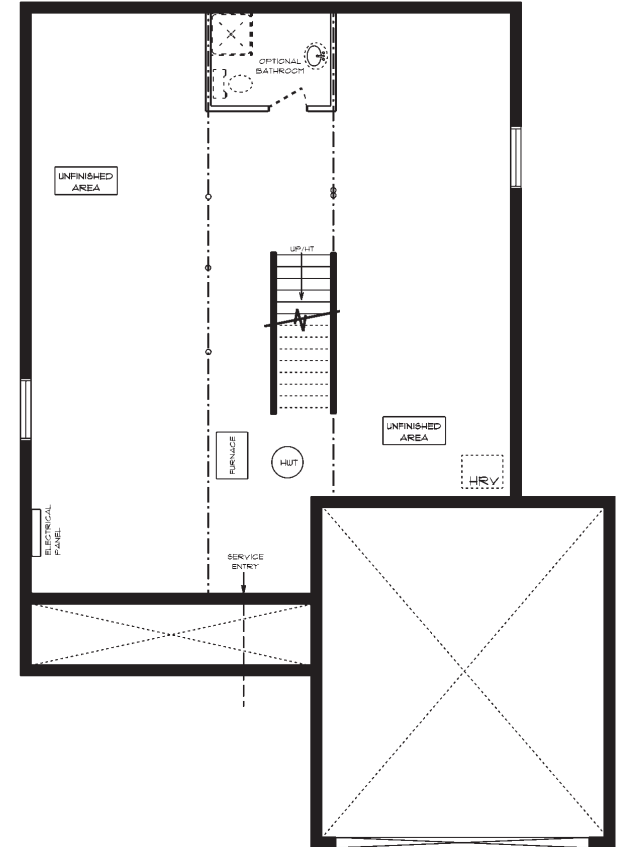
BASEMENT PLAN PLAN DU SOUS-SOL
