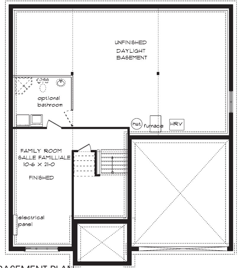
BASEMENT PLAN PLAN DU SOUS-SOL
